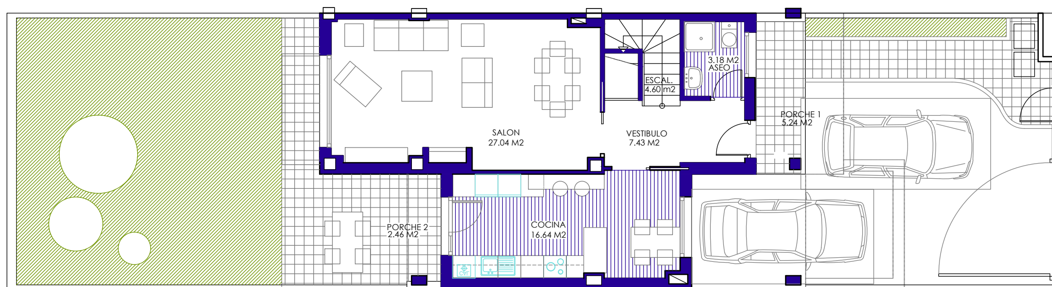
PLANTA BAJA
